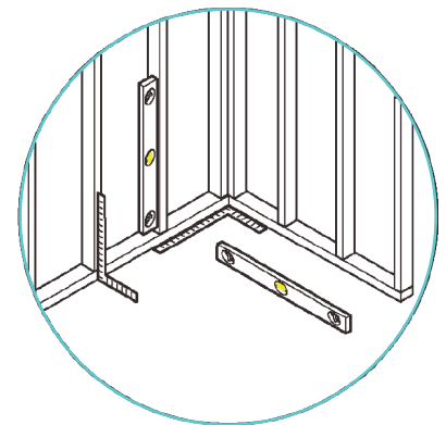
Les montants doivent être affleurants et d'équerre
